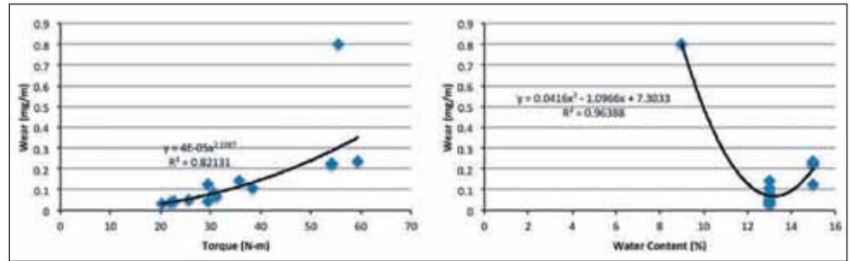
Рис. 8. Влияние крутящего момента и содержания воды на абразивность
