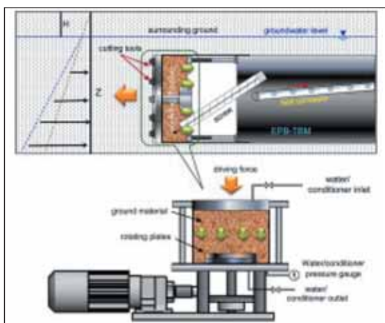
Рис. 6. Камера тестирования абразивности грунта (SATC)
