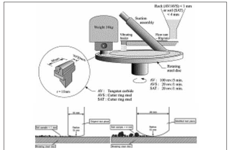
Рис. 4. Испытания методом SAT™
