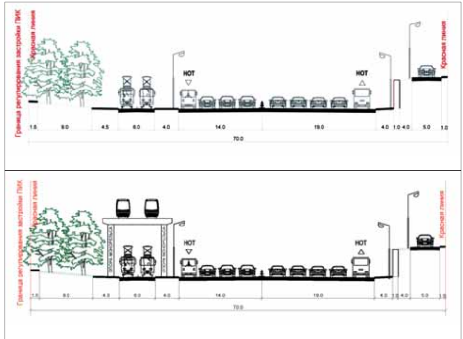
Рис. 2. Существующий и перспективный поперечный профиль Ярославского шоссе в районе ТПУ Росokino при продлении ММТС
