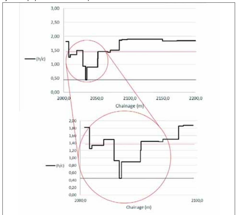
Рис. 9. Текущая потребность в инструменте с точки зрения часов на режущее кольцо шарошки (результаты программного обеспечения)
