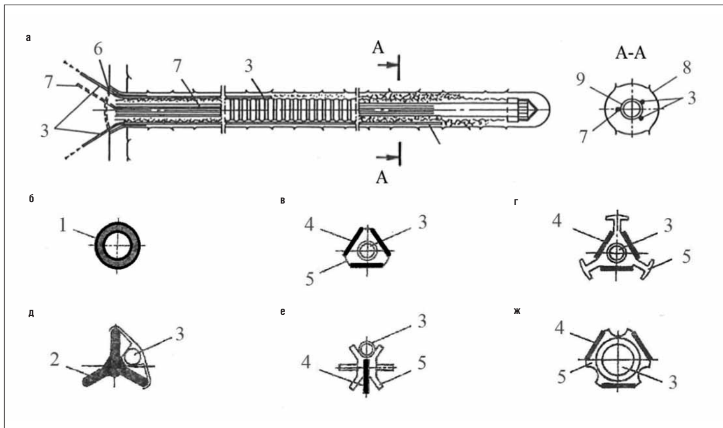
Рис. 2. Конструкция армирующих фибергласовых элементов: а – продольный разрез с поперечным сечением; б–ж – варианты поперечных сечений; 1 – трубчатый элемент; 2 – Y-образный элемент; 3 – трубка для инъектирования; 4 – плоский элемент; 5 – кондуктор; 6 – пробка из расширяющегося пластического материала; 7 – трубка для отвода воздуха; 8 – скважина; 9 – фибергласовая трубка
